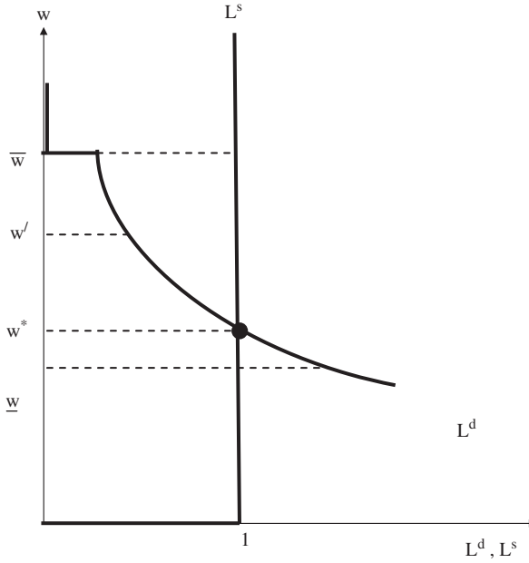
Fig. 1. Unique equilibrium.
